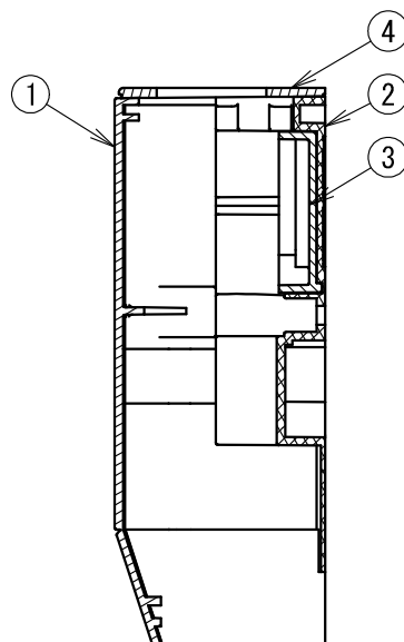
断面 A-A
